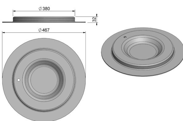
FLANGE 7.14 COM BUJÃO M16X1,5 INFERIOR
