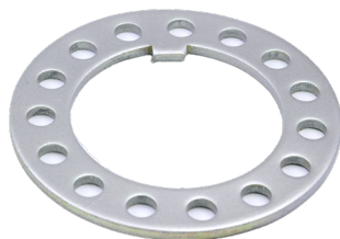
ARRUELA TRAVA CARÇAÇA D60 TINKINHO 5.257.209
